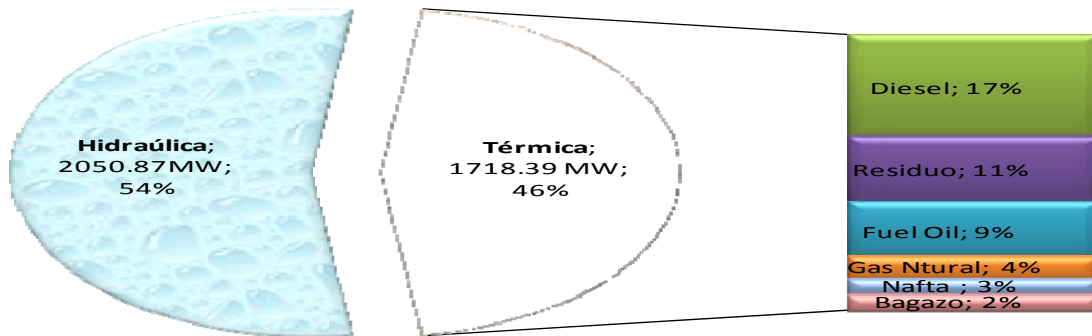
Gráfico 50 Capacidad instalada de generación eléctrica del Sistema Nacional Interconectado (Porcentaje y megavatios)
