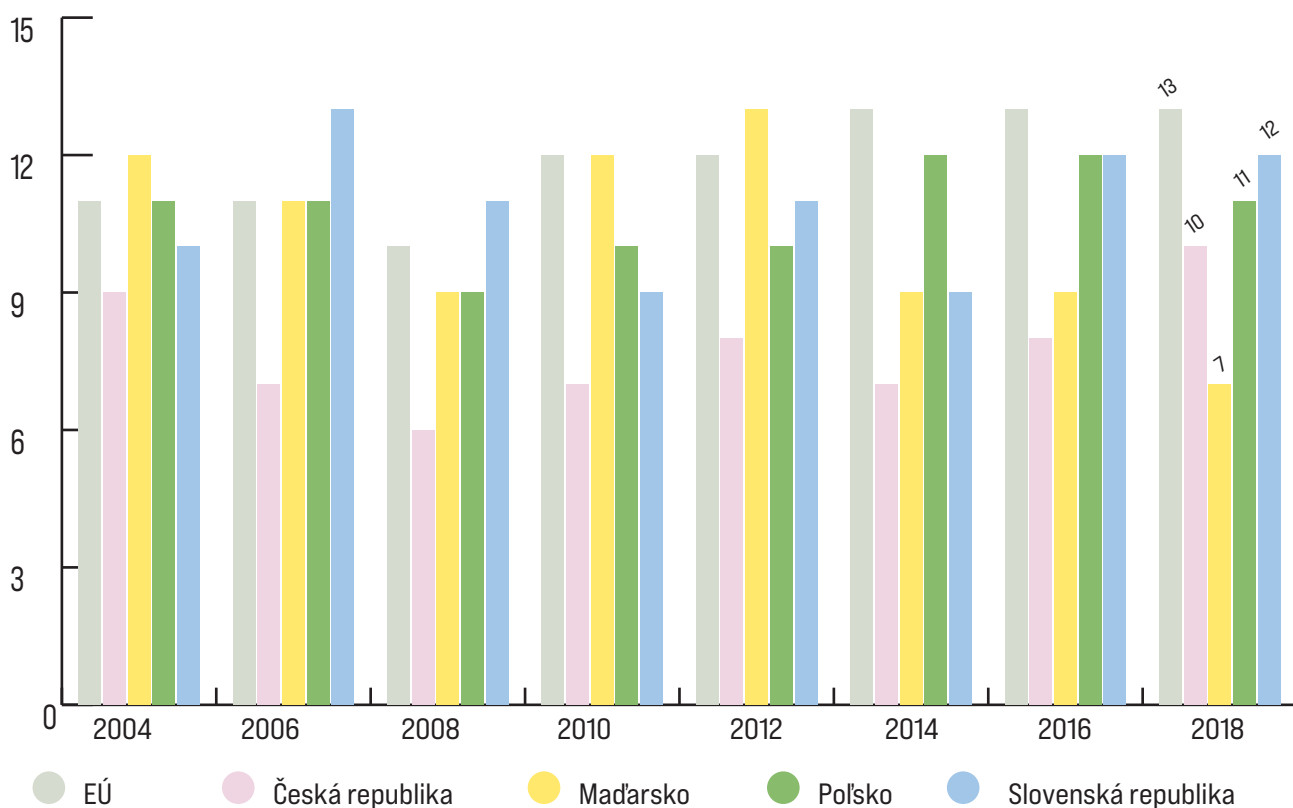
Graf 3 Vývoj tvorby celkového odpadu bez majoritných skupín odpadu z minerálov v krajinách V4 a EÚ v rokoch 2004, 2006, 2008, 2010, 2012, 2014, 2016 a 2018 [% z domácej materiálovej spotreby]
