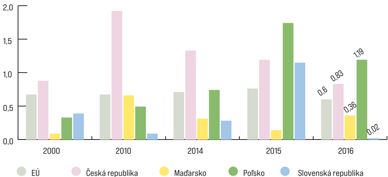
Graf 12 Vývoj počtu podaných patentov súvisiacich s recykláciou a spracovaním druhotných surovín v krajinách V4 a EÚ v rokoch 2000, 2010 a 2014-2016 (na mil. obyv.)
