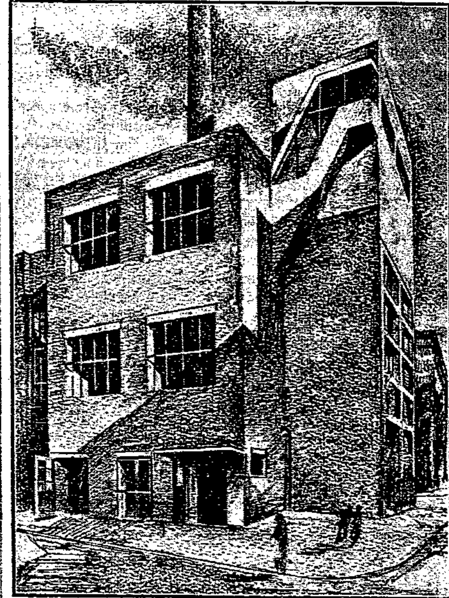
Das neue Maschinenhaus des Konsumvereins Magdeburg.
