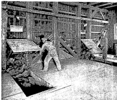
Einwurftrichter der Vorbrecher, die aus den mit Rohgestein gefüllten Vorbunkern beschickt werden.
