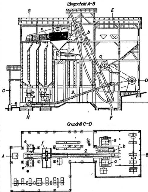
Eine neuzeitliche Schotter- und Splittbereitungsanlage im Schnitt.
