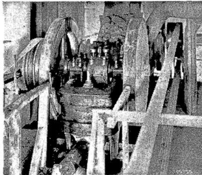
Nachbrecher zur Herstellung von Kleinschotter.
