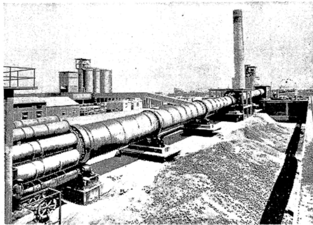
Ein 90 m langer Zement-Brennofen In der umlaufenden eisernen Röhre wird das nasse Gemisch aus gemahlenem Kalkstein und Ton zu Klinkern gebrannt. Am Auslaufende des Ofens sind kreisförmig 12 Käl- deröhre angeordnet, in denen die gebrannten Klinker abgeköhlt werden
