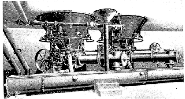
Homogenisator Diese Einrichtung dient zur innigen Mischung der für die Zementherstellung erforder- lichen Rohstoffe, die vor dem Brennen fein vermahlen und möglichst gleichmäßig mit- einander vermengt werden müssen, damit der fertige Zement immer die gleichen Eigen- schaften aufweist
