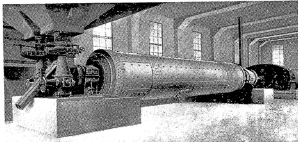
Zementmühle, In der die in den Oefen gebrannten Klinker staubfein zermahlen werden
