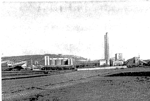
Gesamtansicht einer neuzeitlichen Portlandzementfabrik, in der täglich etwa 500 t Zement hergestellt werden können
