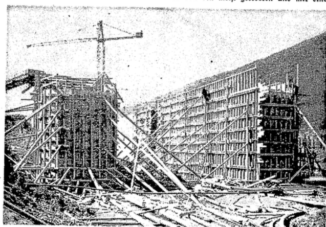
Einschalung des Schleusenunterhauptes und des Schleusenpfeilers.
