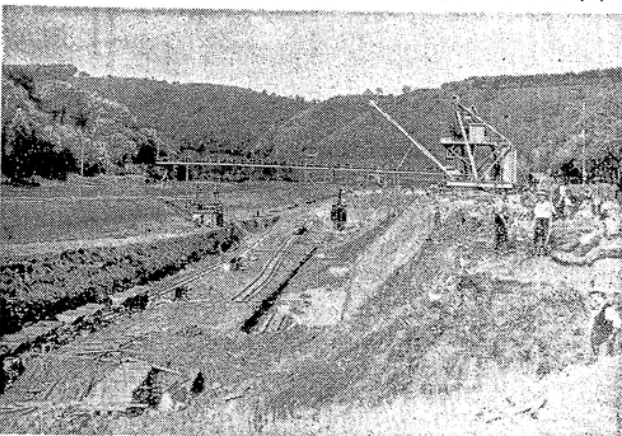
Schleusenbaugrube vor Beginn der Betonarbeiten.
