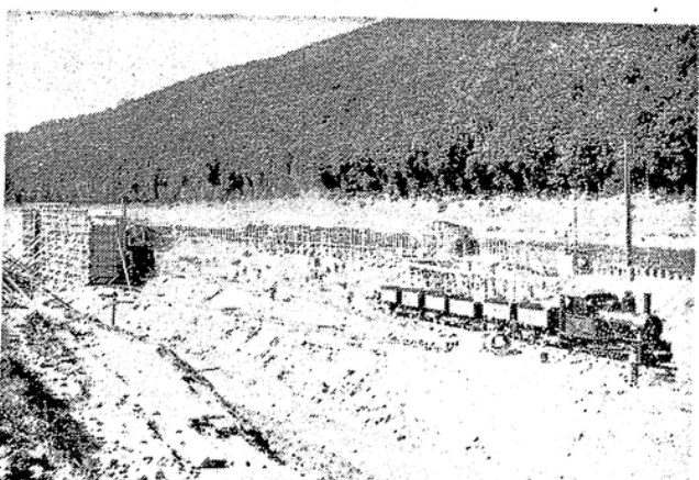
Baugrubenumschließung für die rechte Wehröffnung und Aushub für die Wehrsohle.
