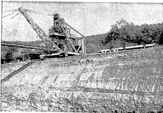
10 m hohe Böschung der Schleusenammern und Betoniermaschine.
