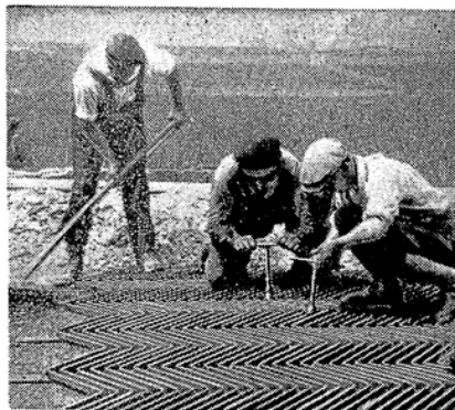
Herstellung der Schraubenverbindung zwischen den einzelnen Elementen der Rostdecke.
