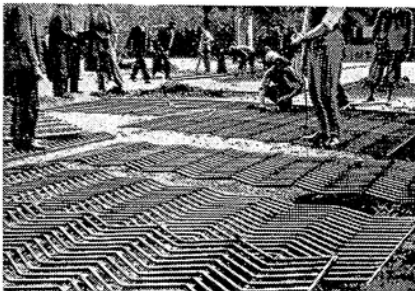
Zusammenbau der Rostelemente.
