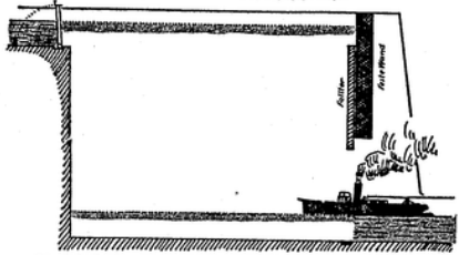
Die Schiffschleuse des Winden am Weste-Ost-Kanal hat 85 Meter Schluslänge, 10 Meter Breite und 15 Meter Höhe.
