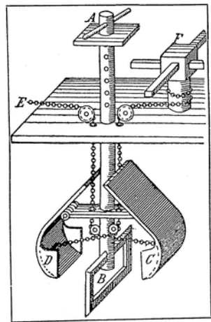
Dampfbagger von 1867, nach der Art der jetzigen Greifbohrer gebaut.
