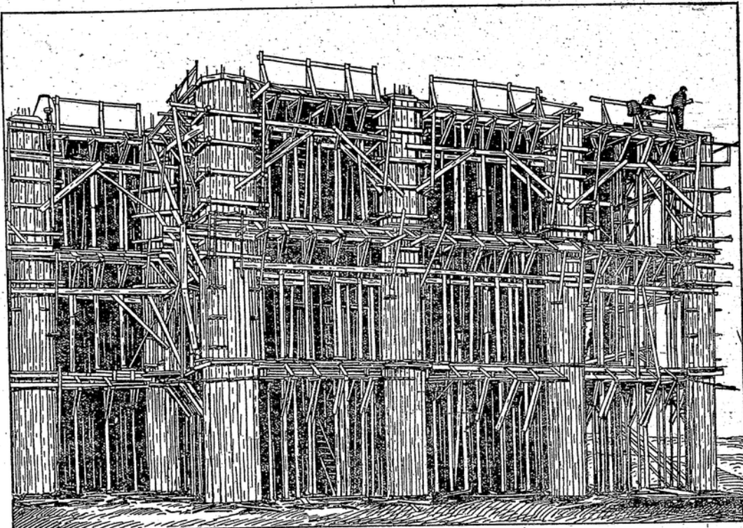
Eisenbetonbau in Berlin-Tempelhof 1912.
