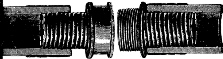
Abb. 17. Pretzel's Schlauch-Verschraubung.
