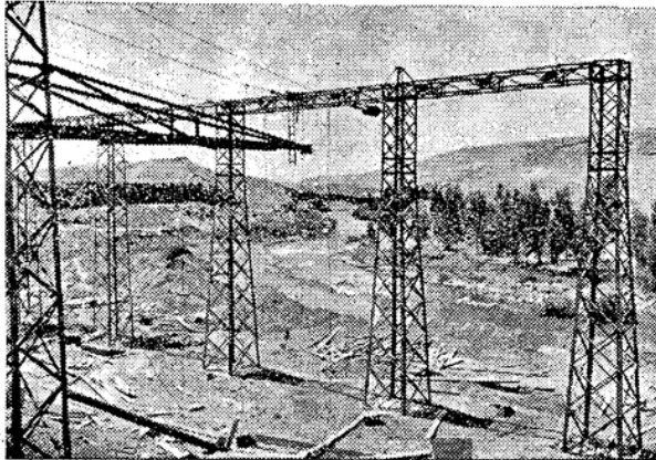
Transformatorbau neben der zentralen Kraftstation am Jordan.
